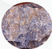
تراکیت آندزیت داسیت
